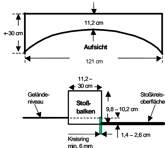
Stoßbalken nach IAAF - Spezifikation
